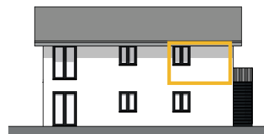
Ostansicht
